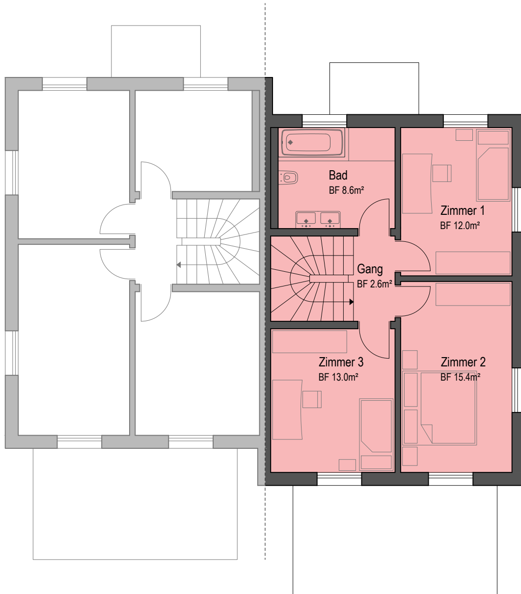
Obergeschoss Haus 5
