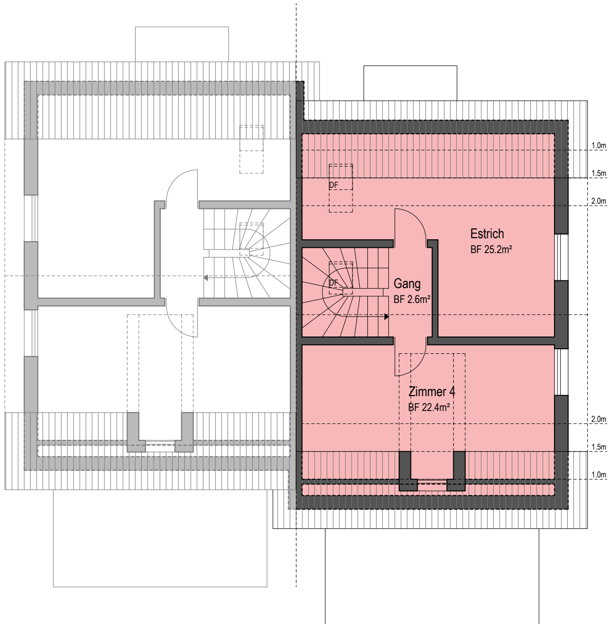
Dachgeschoss Haus 5
