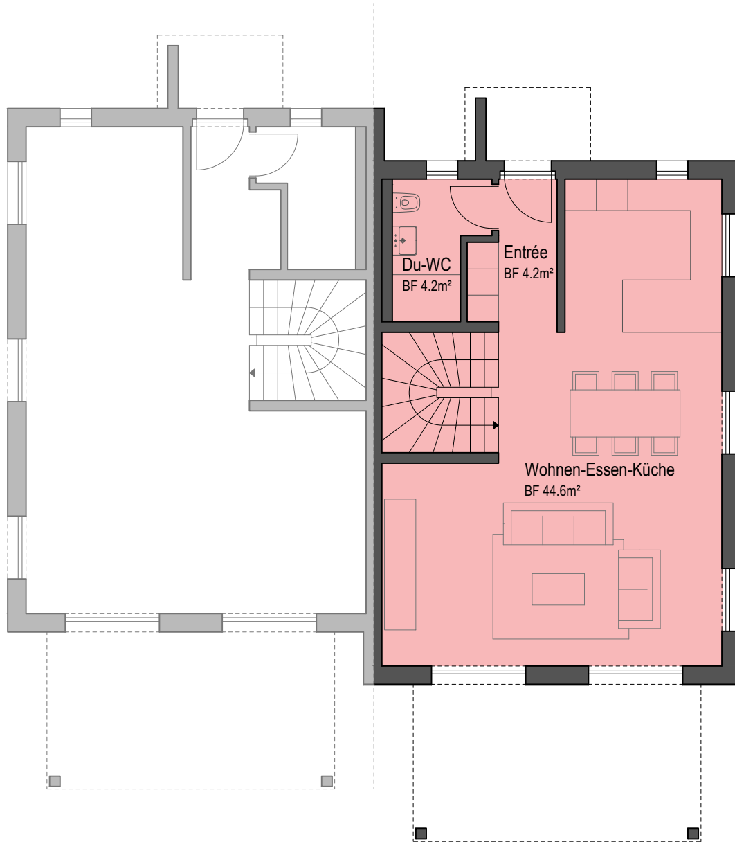
Erdgeschoss Haus 5
